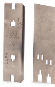
ШАБЛОН ДЛЯ ЗАТОЧКИ 3/8" NOBBY 505 69 81-03
